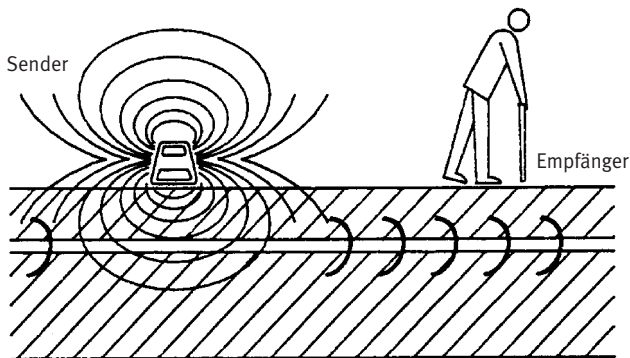
Bild 7: Aktives Orten mit Hilfe eines Senders und eines Empfängers
